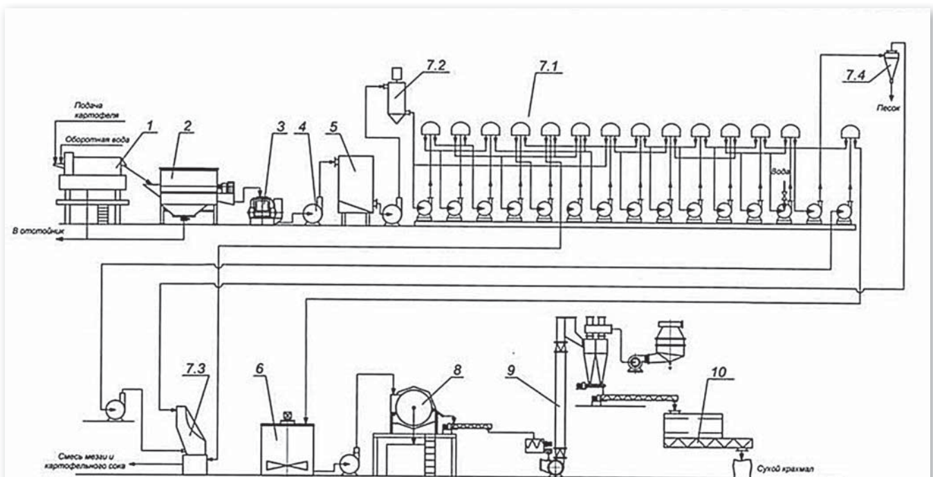
Технологическая схема переработки картофеля мощностью 200 т/с
